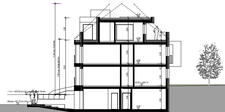
querschnitt 1:100
