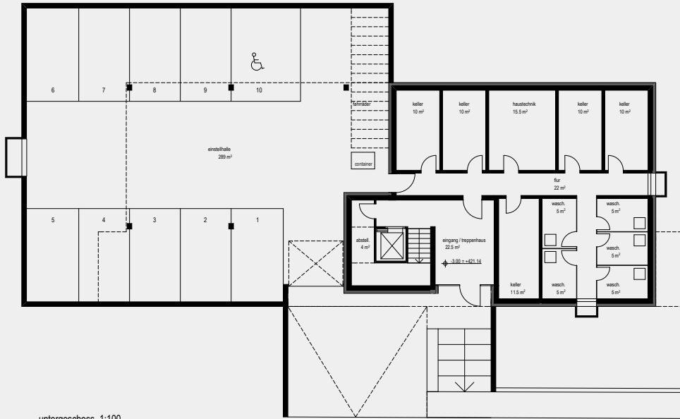
untergeschoss 1:100
