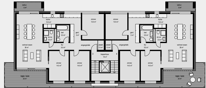
obergeschoss 1:100
