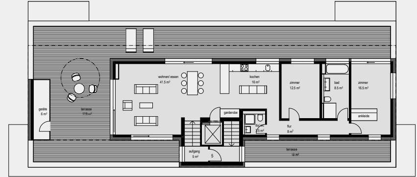
dachgeschoss 1:100
