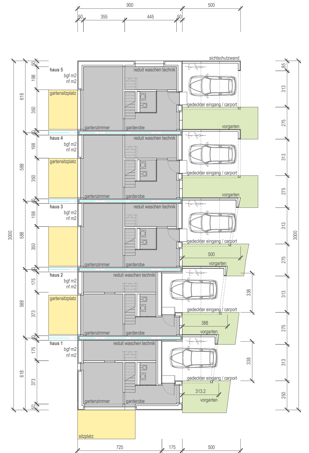
erdgeschoss
