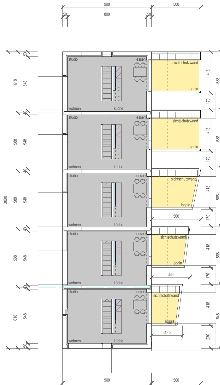
obergeschoss
