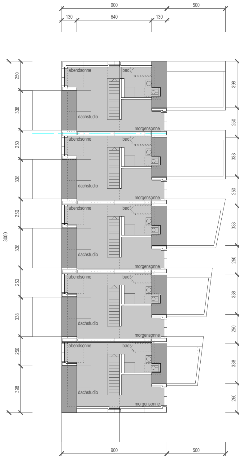
dachgeschoss
